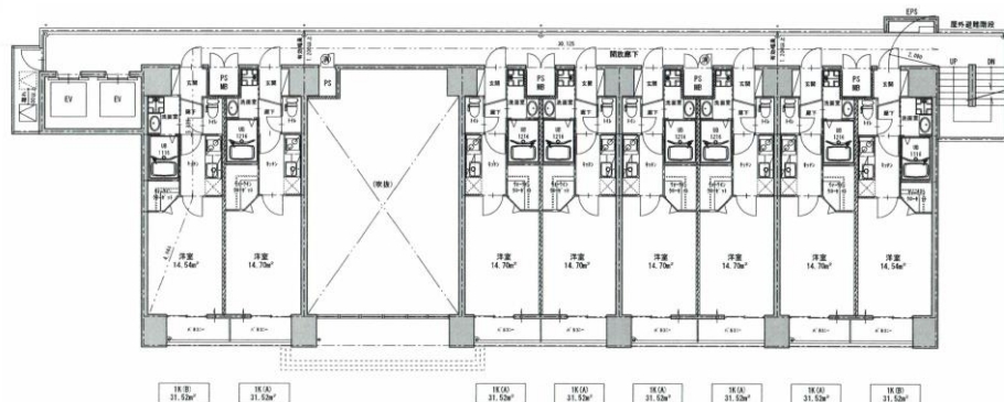
2階平面図
